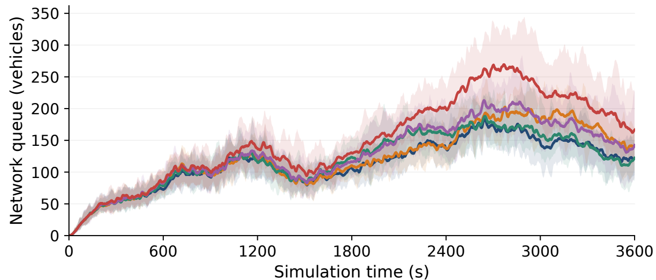
IQLL
