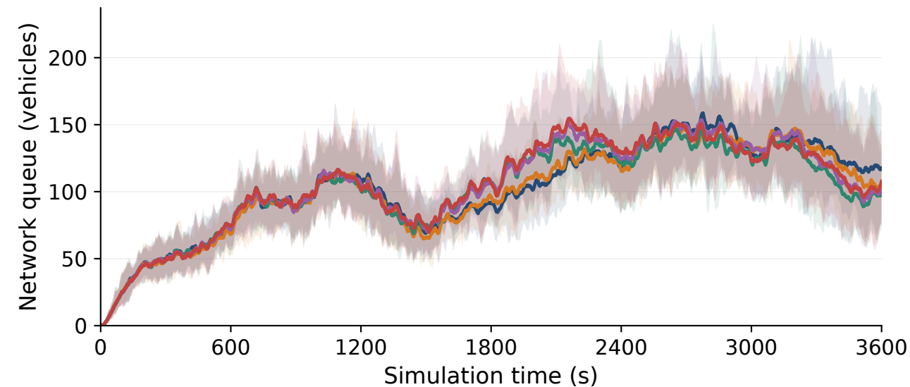
PPO
